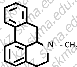
Апорфин
