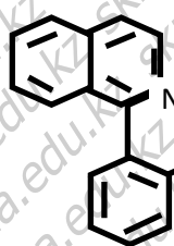
Бензилизохинолин
