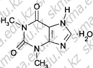
Теofilлин-Theophyllum. 1,3-Диметилксантин.
