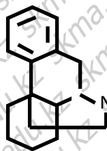
Морфинан
