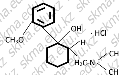
Трамал (±)-Транс-2-[диметил-
